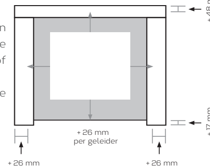
Type 2 "In de Dag"
