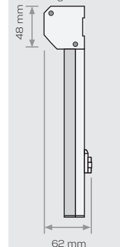
Type 3 "In de Dag" Bedieningsrail tov de cassette gedraaid.
