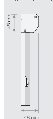
Type 1 "Op de Dag"
