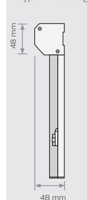
Type 2 "In de Dag"
